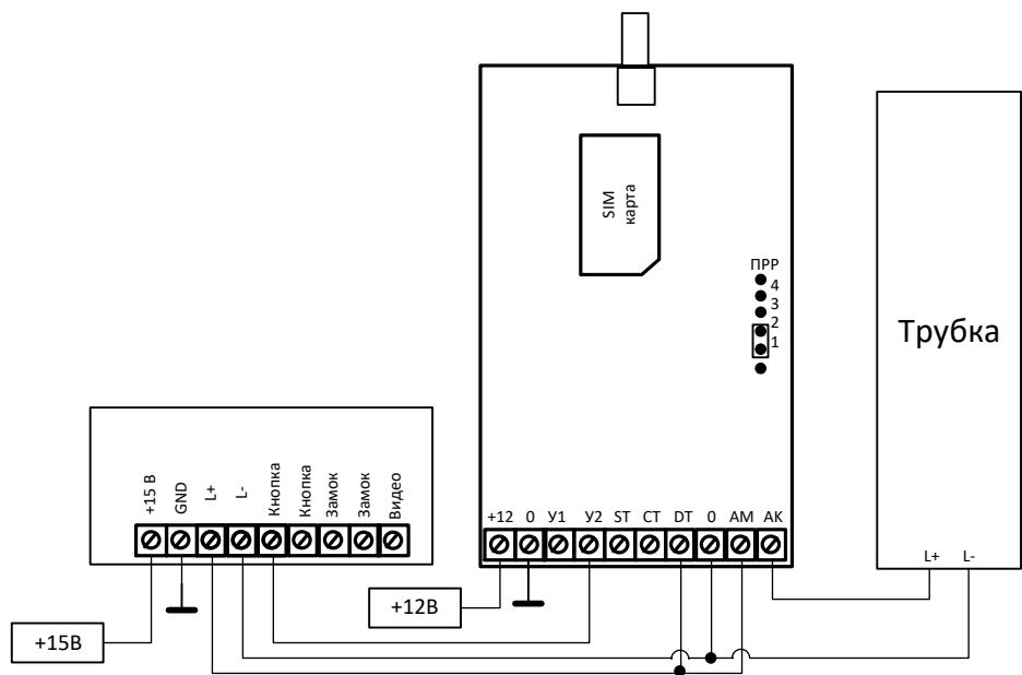
Подключение приставки
