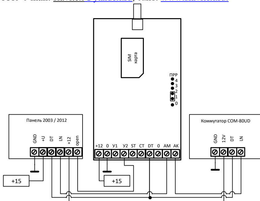
Схема подключения с коммутатором
