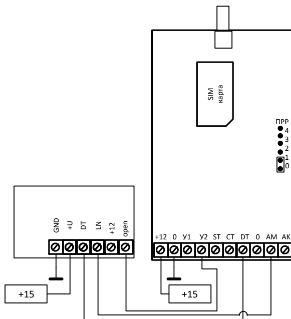
Схема подключения без коммутатора
