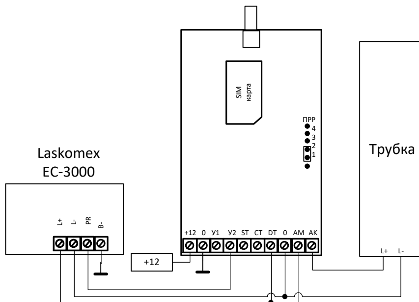
Рис. 1. Подключение приставки
